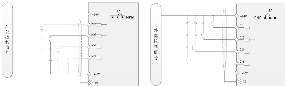
a. NPN 型接线方式
