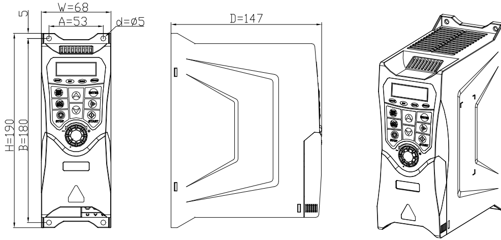
图 3.1 外形及壁挂式安装尺寸示意图
